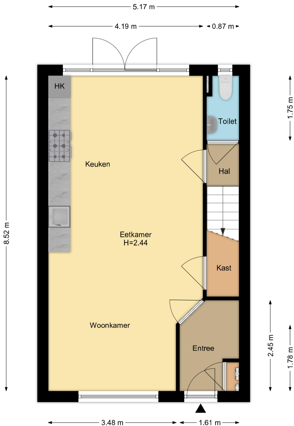
Begane Grond Malthusstraat 1, Haarlem R.M. Vastgoedpresentatie| Aan deze plattegrond kunnen geen rechten worden ontleend
