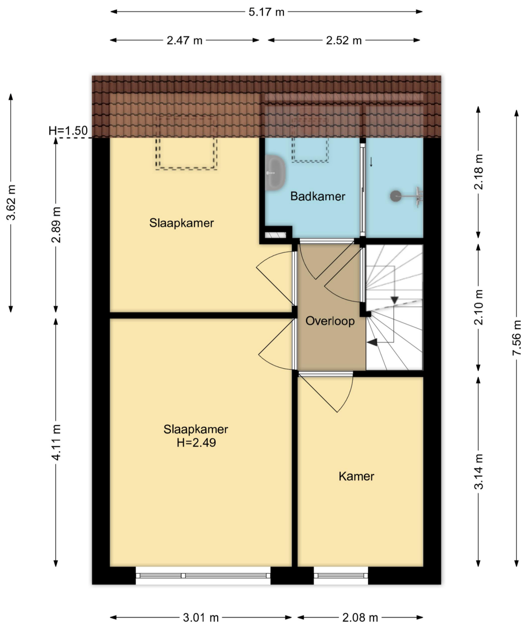
1e Verdieping Malthusstraat 1, Haarlem
