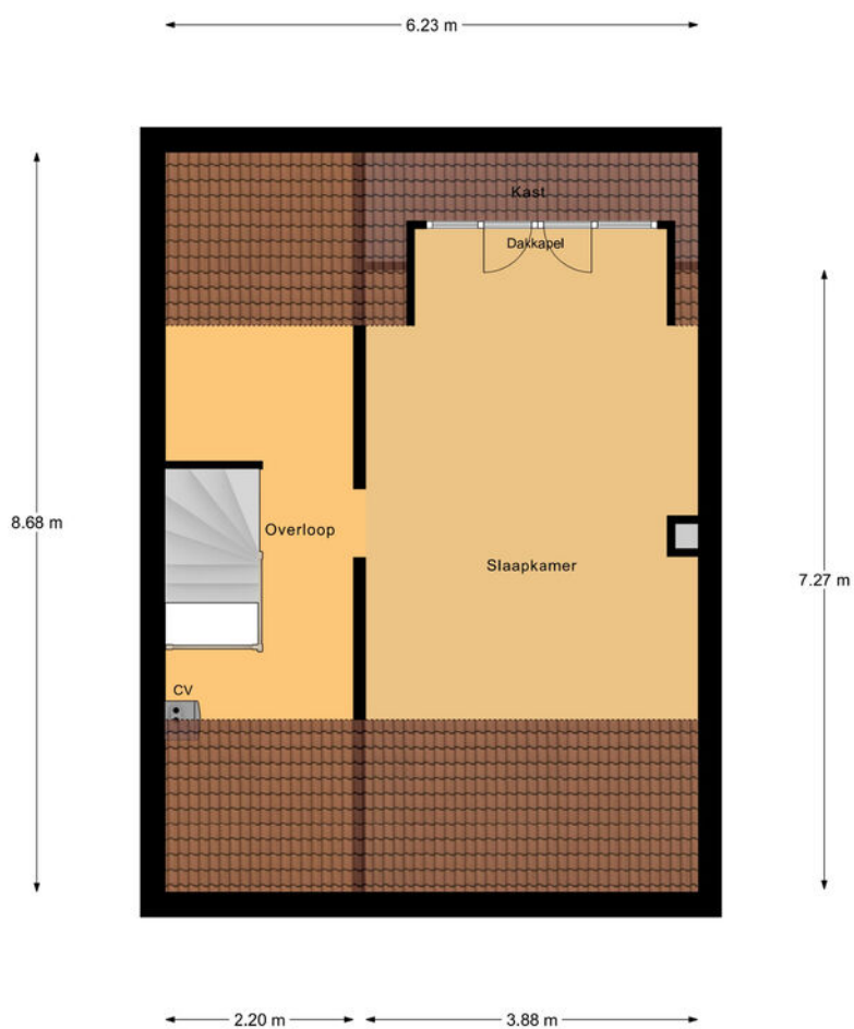
2e Verdieping
