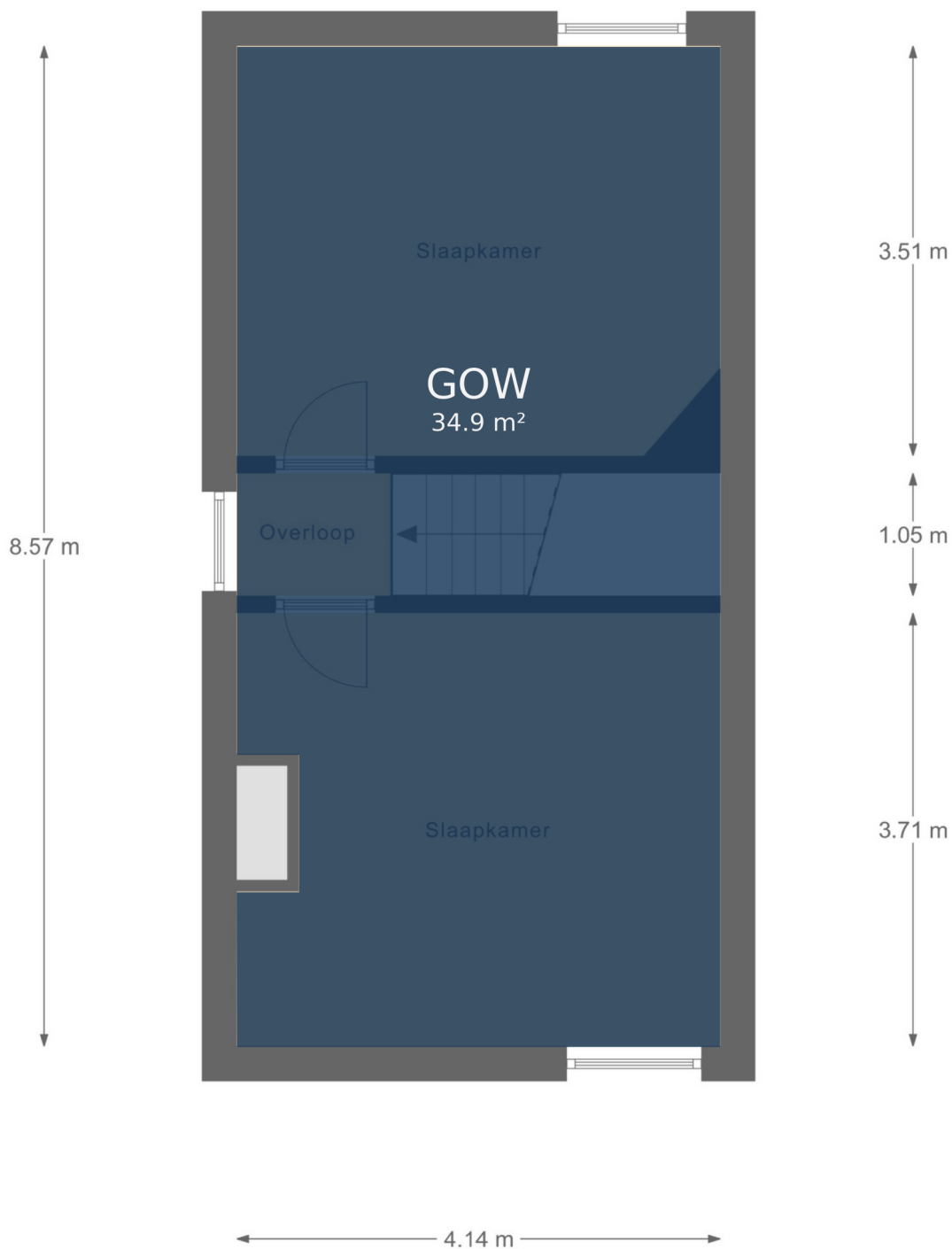
1e Verdieping
