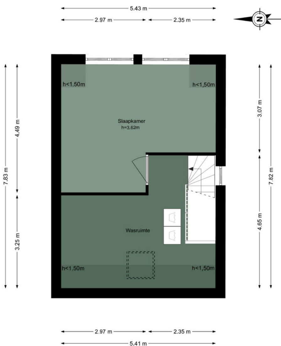
Floris V Dreef 46 - Blaricum Tweede verdieping
