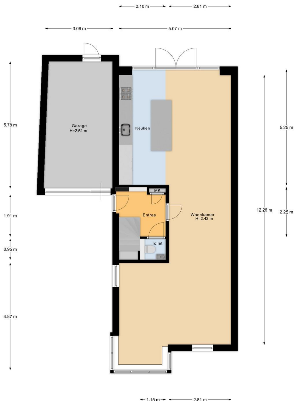
Begane Grond
