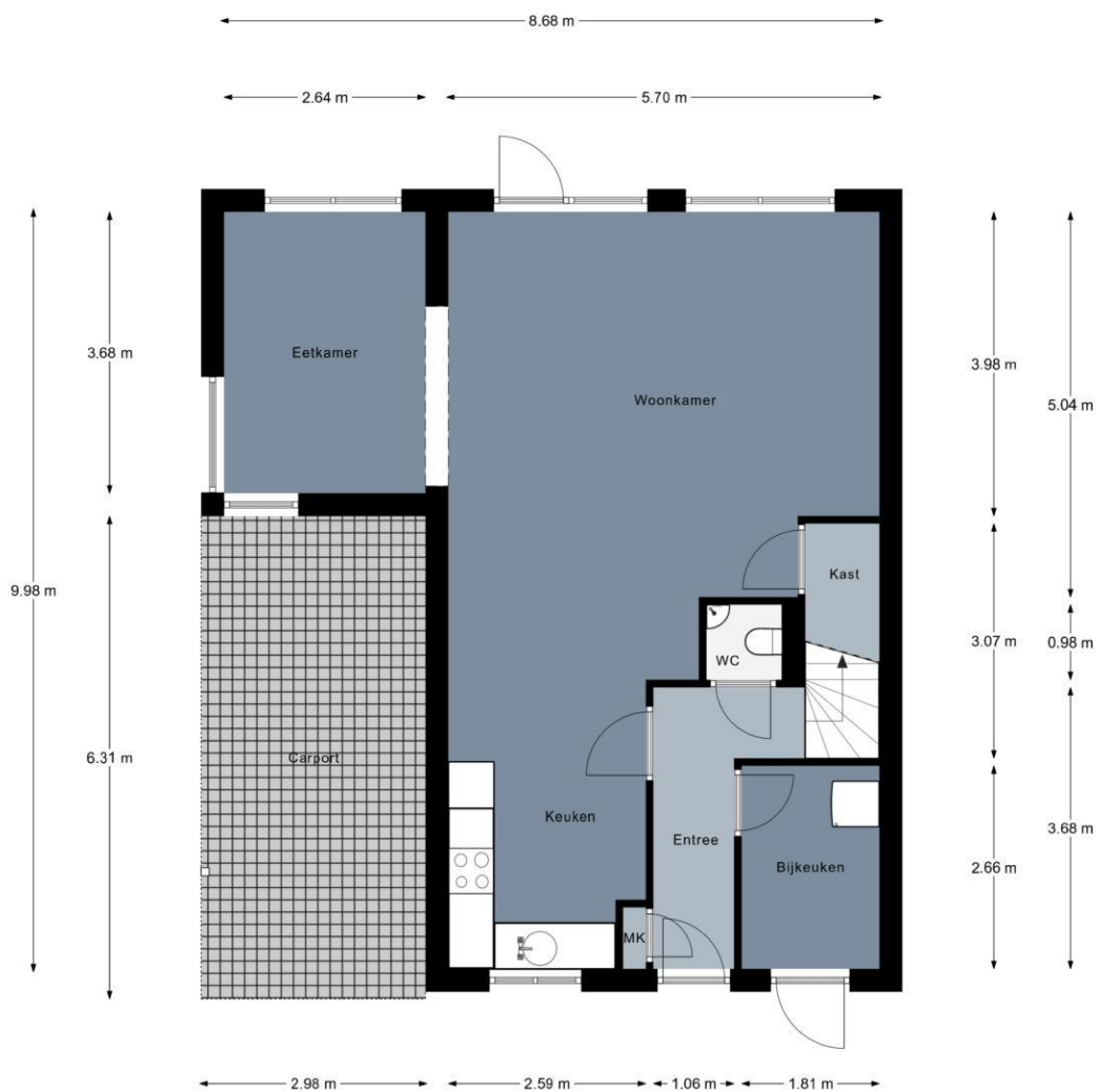
Begane Grond
