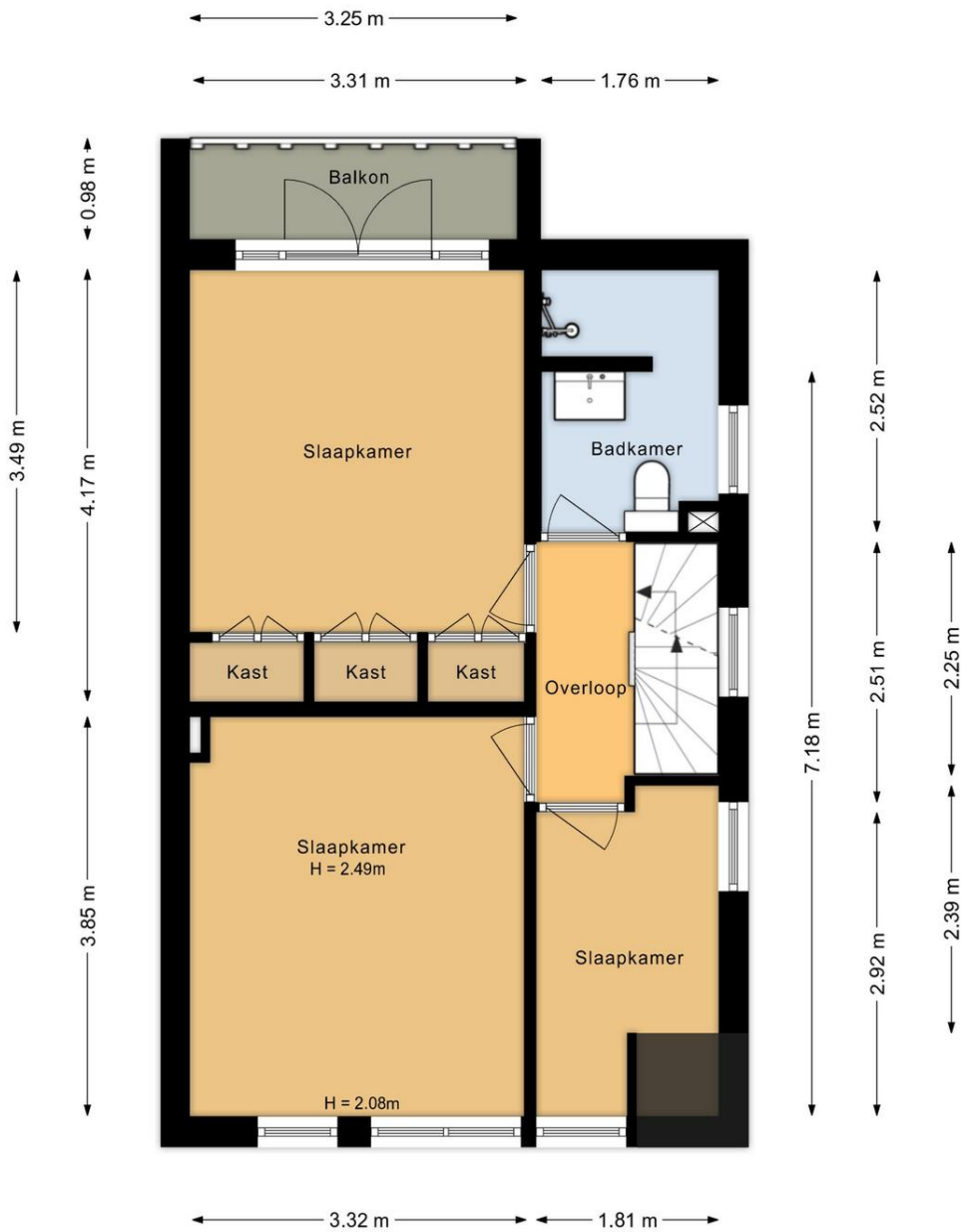
Eerste verdieping Lambrecht van Dalelaan 33 Haarlem
