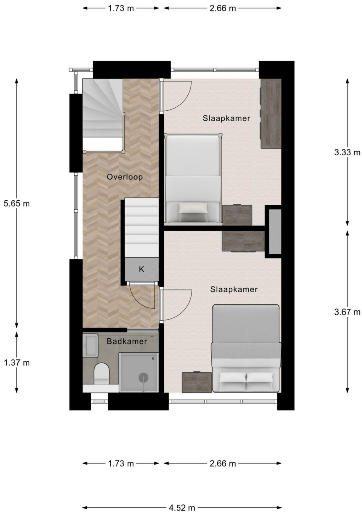
1e Verdieping
