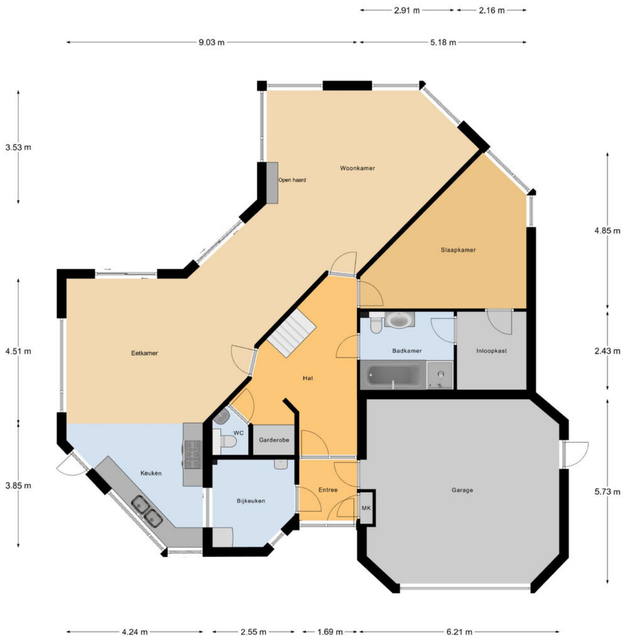
Begane Grond
