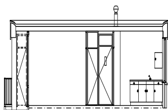
Doorsnede
