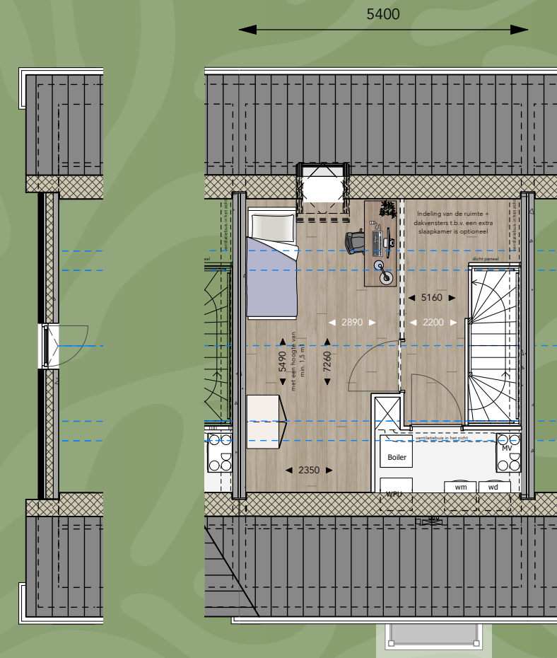
BOUWNR. 68 LINKER ZIJEVEL
