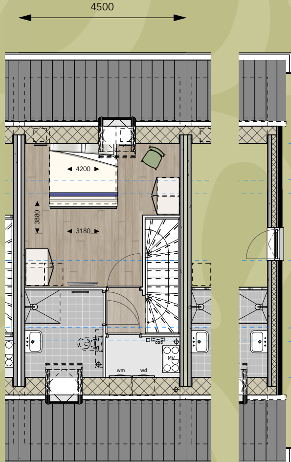
INDELING 2 (afhankelijk van bouwnummer als getekend of gespiegeld)
