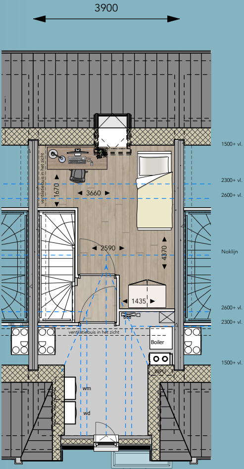
BOUWNR. 2, 8, 33, 39, 43, 48 (afhankelijk van bouwnummer als getekend of gespiegeld)
