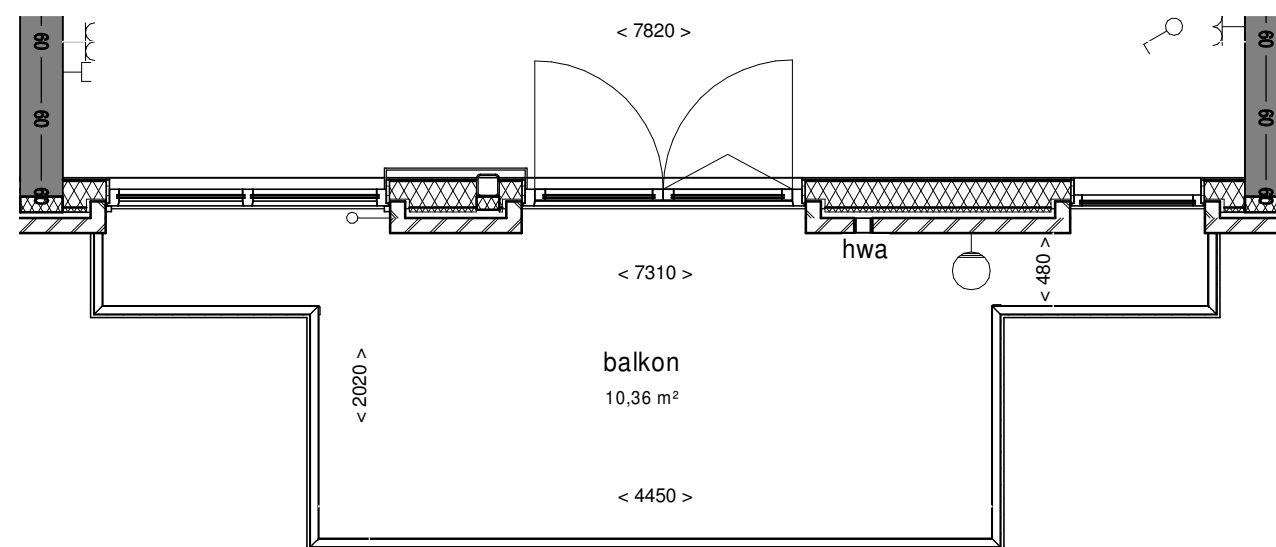
westgevel Bouwnrs.: 02.19/04.19
