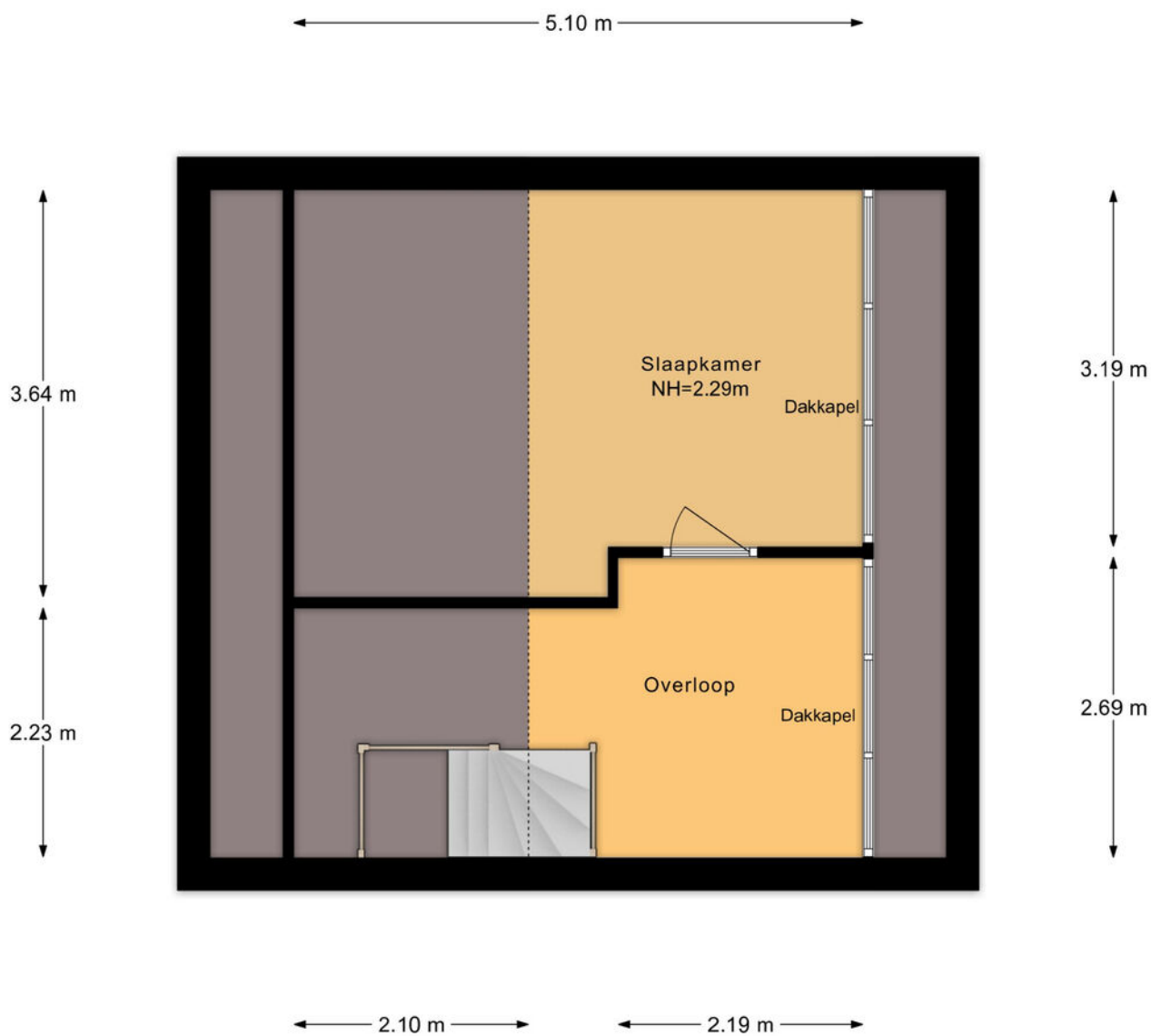
2e Verdieping
