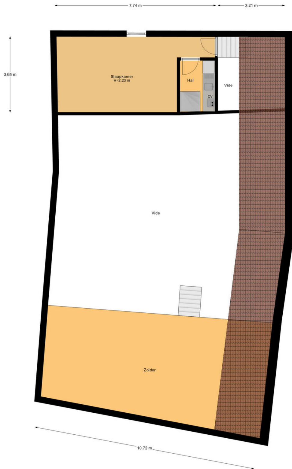
1e Verdieping
