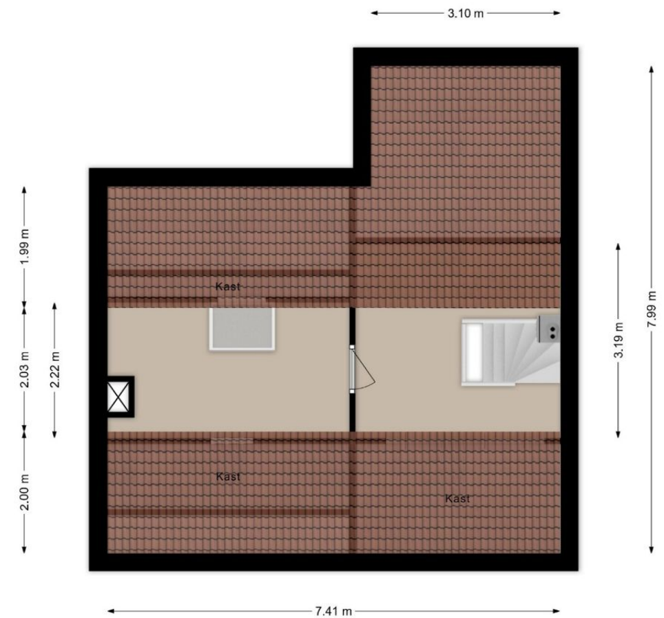
Plattegrond tweede verdieping Aan deze tekening kunnen geen rechten worden ontleend
