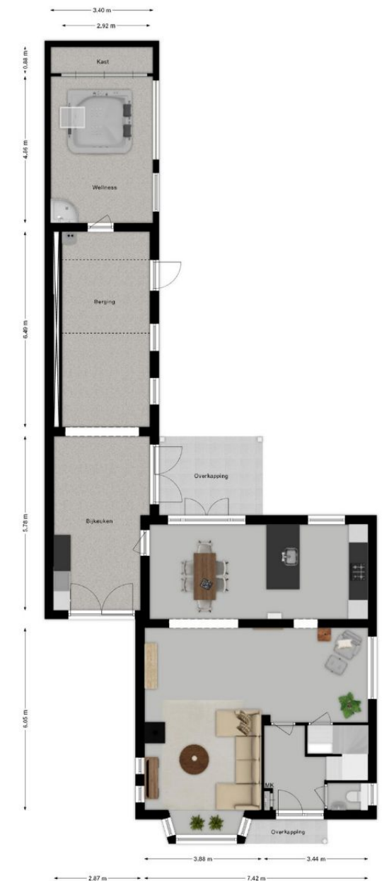
Plattegrond begane grond Aan deze tekening kunnen geen rechten worden ontleend
