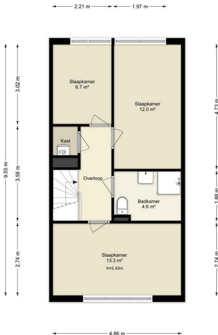
Aartsbisschop Romerostraat 507 - Utrecht Eerste Verdieping
