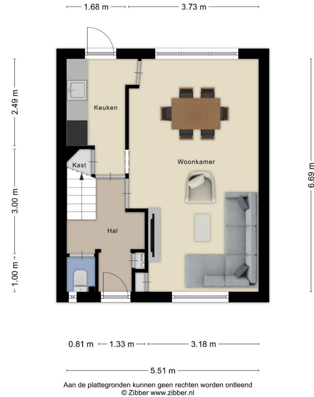
Plattegrond
