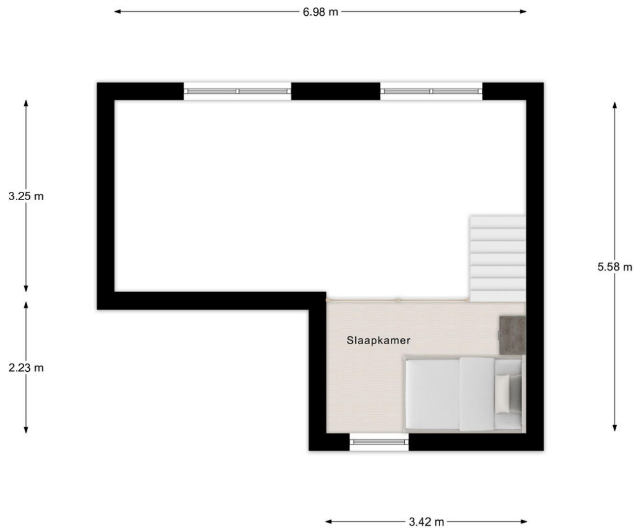
Verdieping 2
