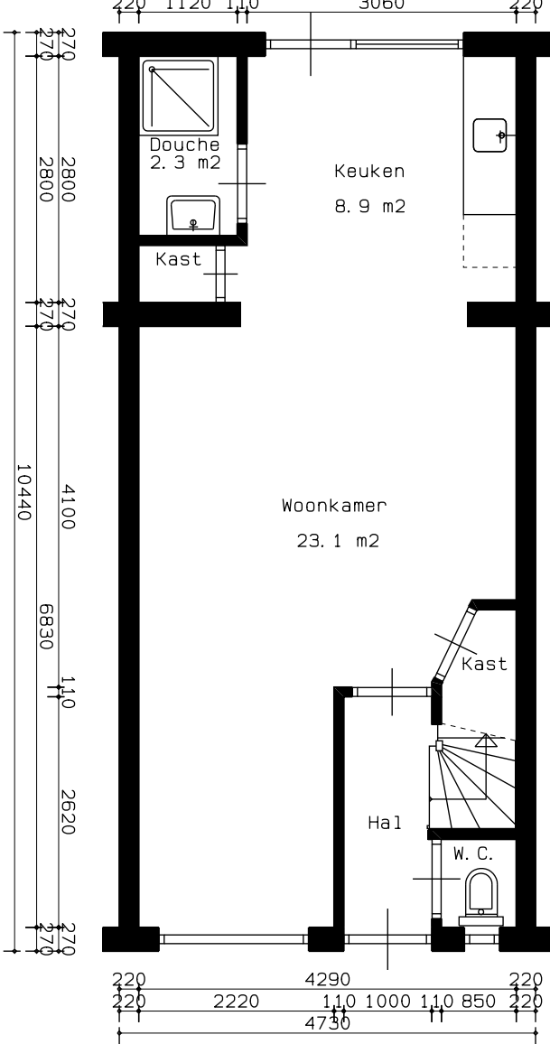
Begane grond
