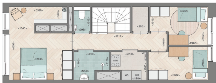
EERSTE VERDIEPING
