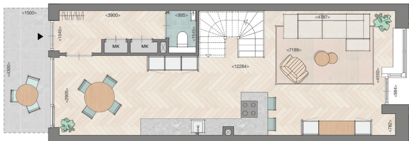
BEGANE GROND
