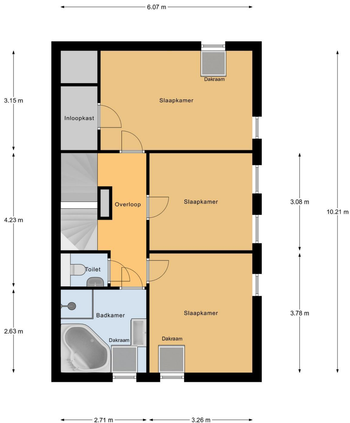
1e Verdieping
