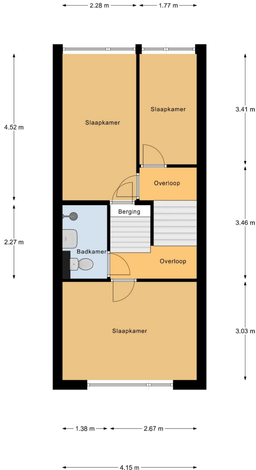
2e Verdieping
