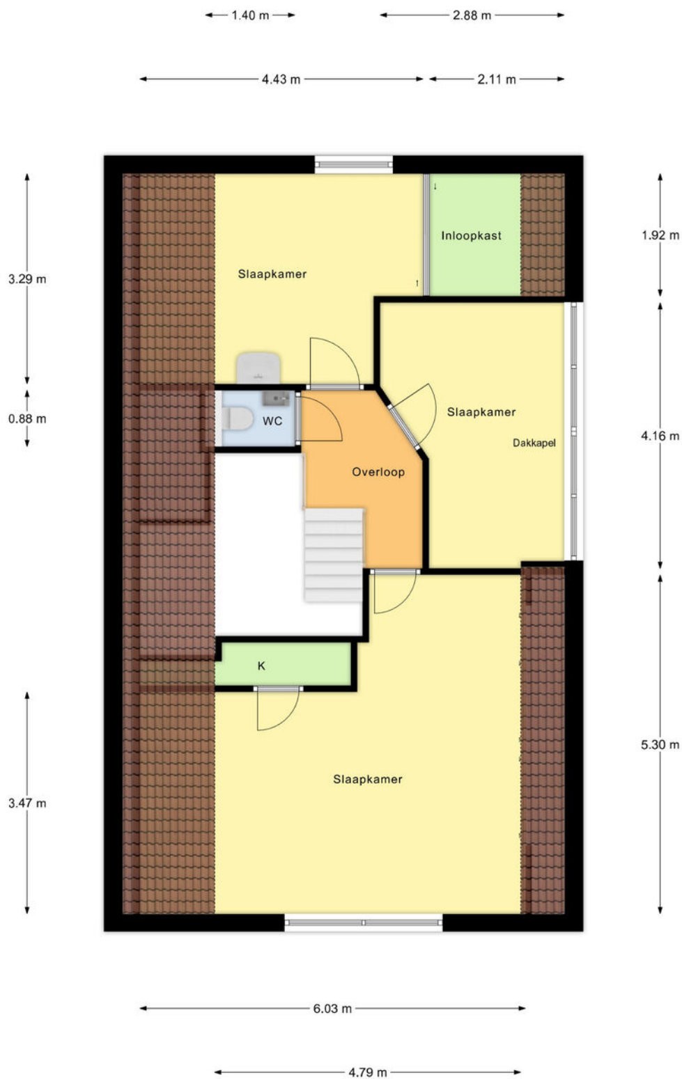
1e Verdieping
