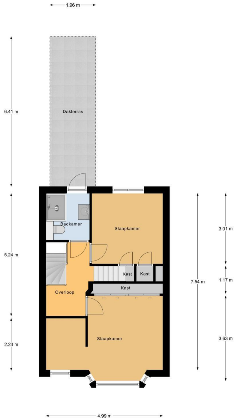
1e Verdieping
