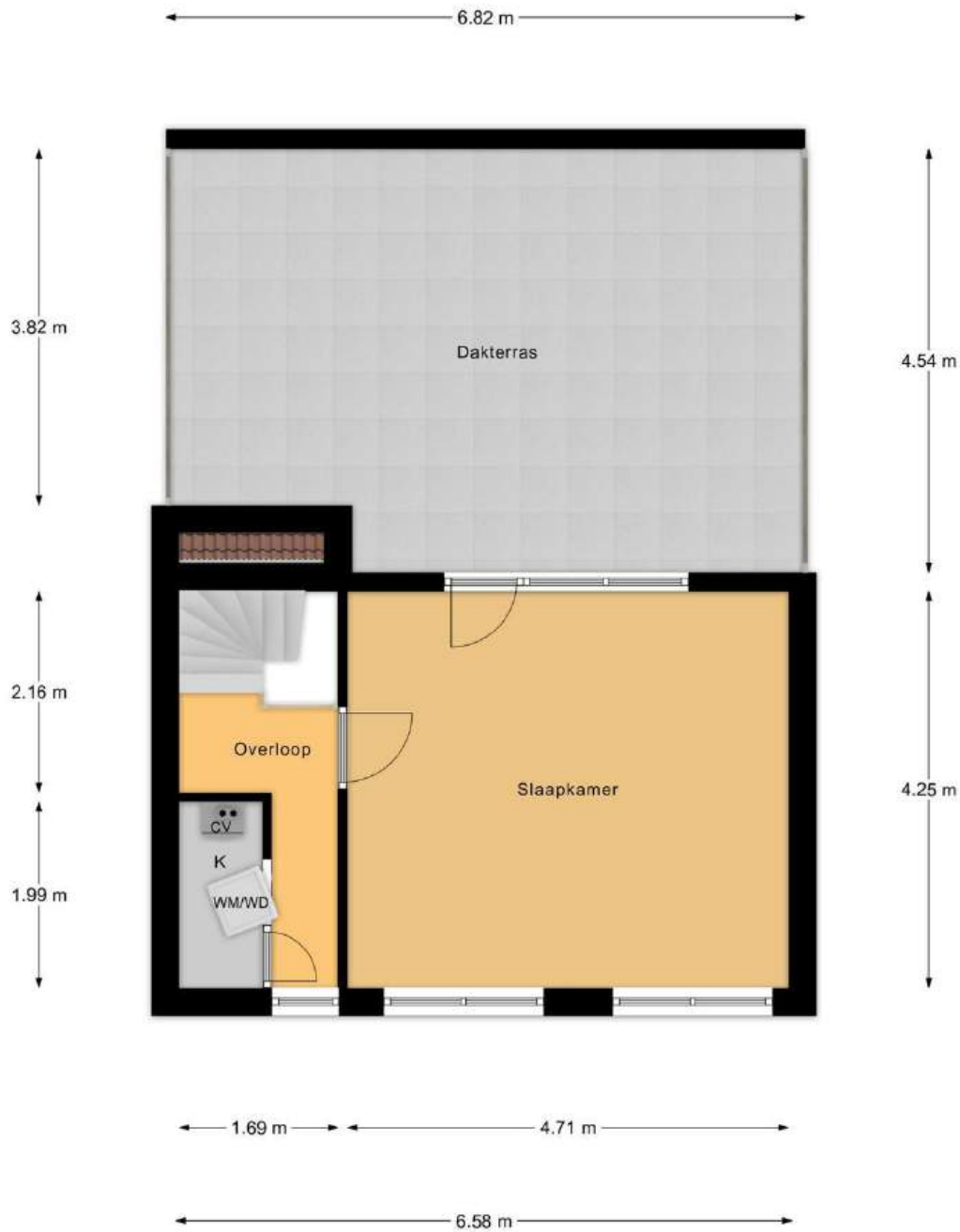
2e Verdieping
