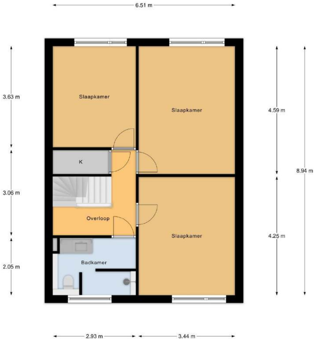
1e Verdieping
