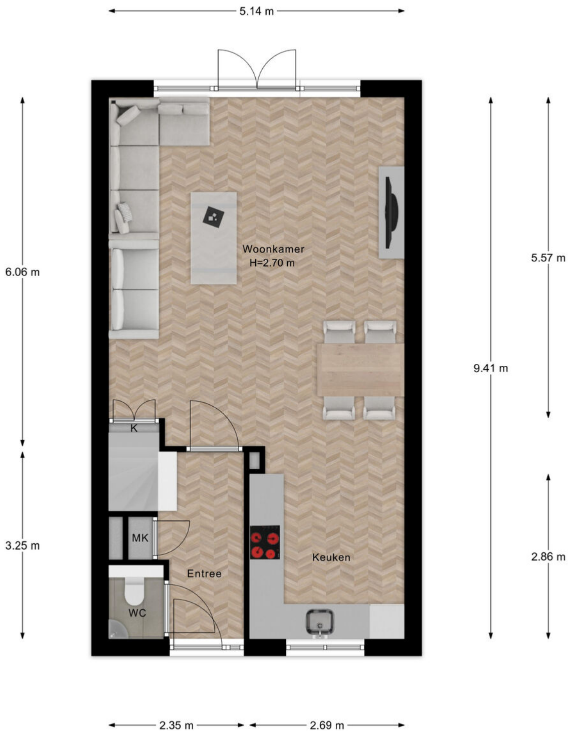
Begane Grond
