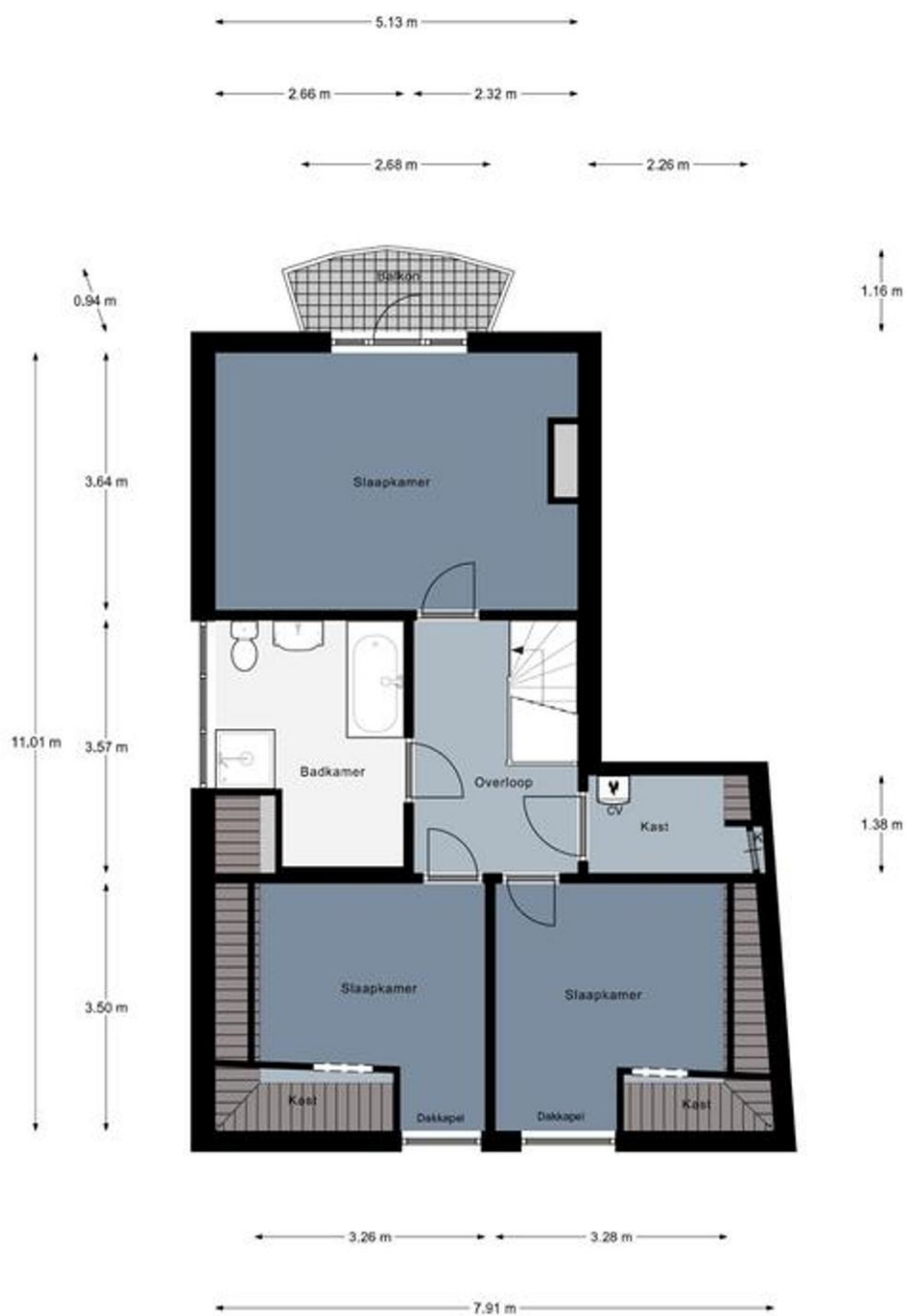
2e Verdieping
