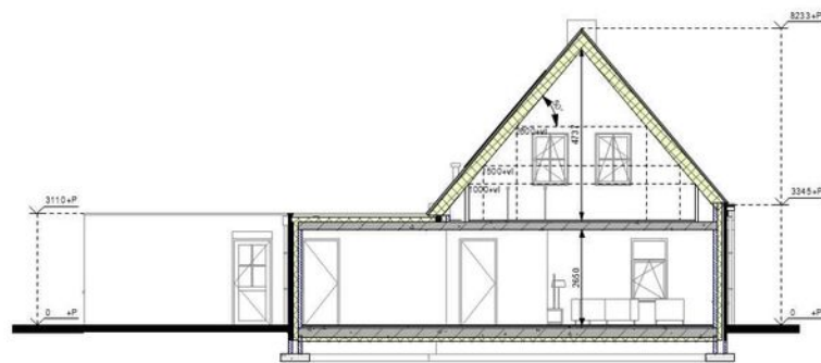
Doorsnede A-A
