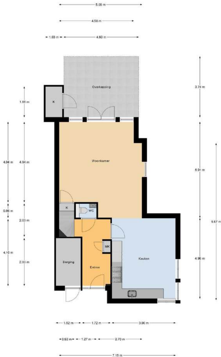
Begane Grond
