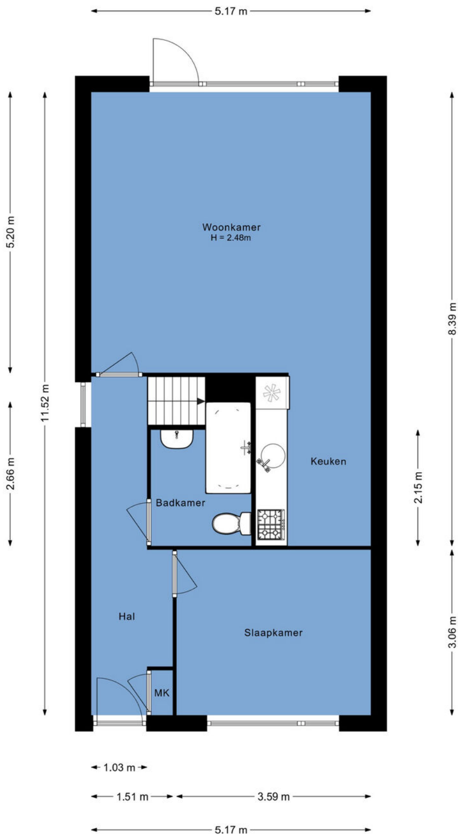
Begane grond Lemenburg 38 Hoofddorp
