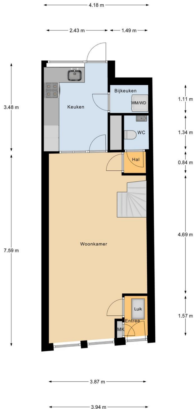
Begane Grond
