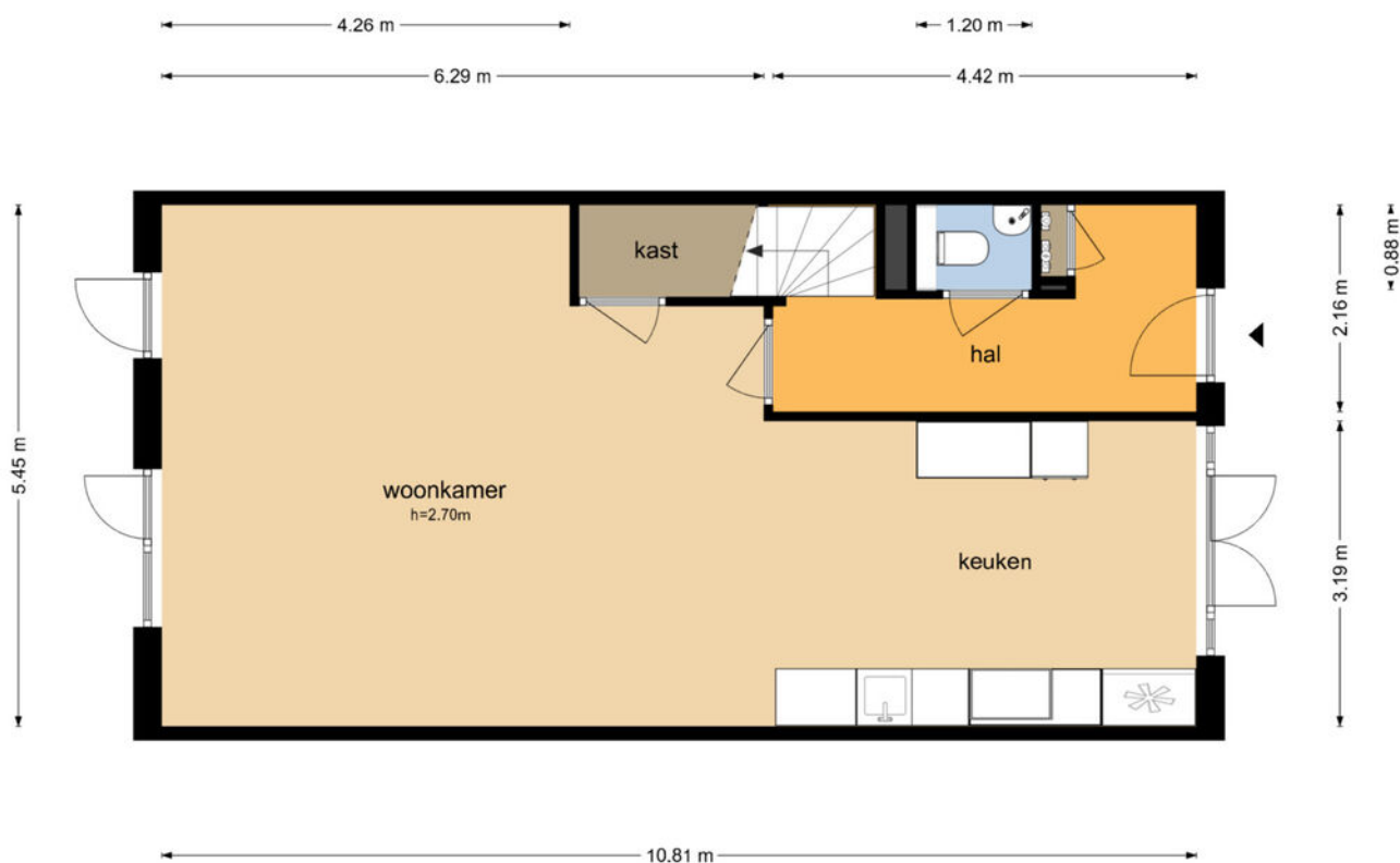
Moutmolen 3 - Delft Begane Grond
