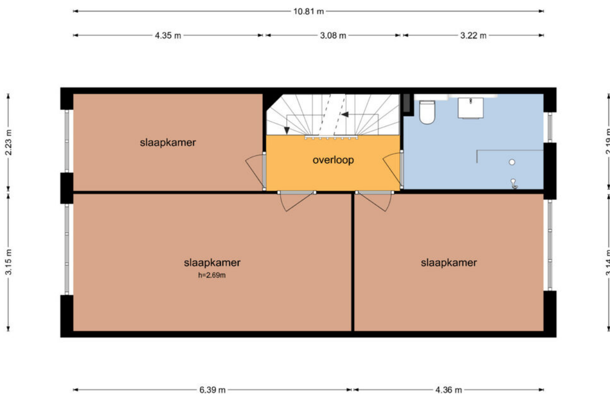
Moutmolen 3 - Delft Eerste Verdieping
