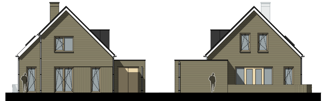
VOORGEVEL (WESTKANT)
