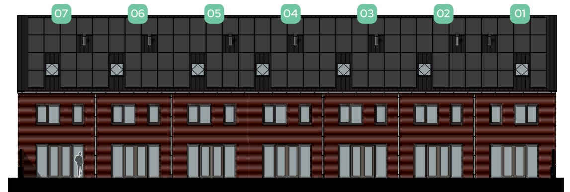
ACHTERAANZICHT ZUIDGEVEL
