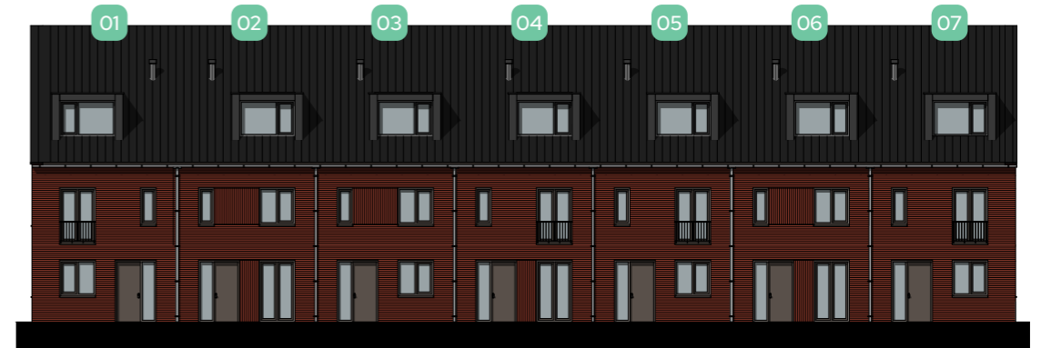
VOORAANZICHT NOORDGEVEL
