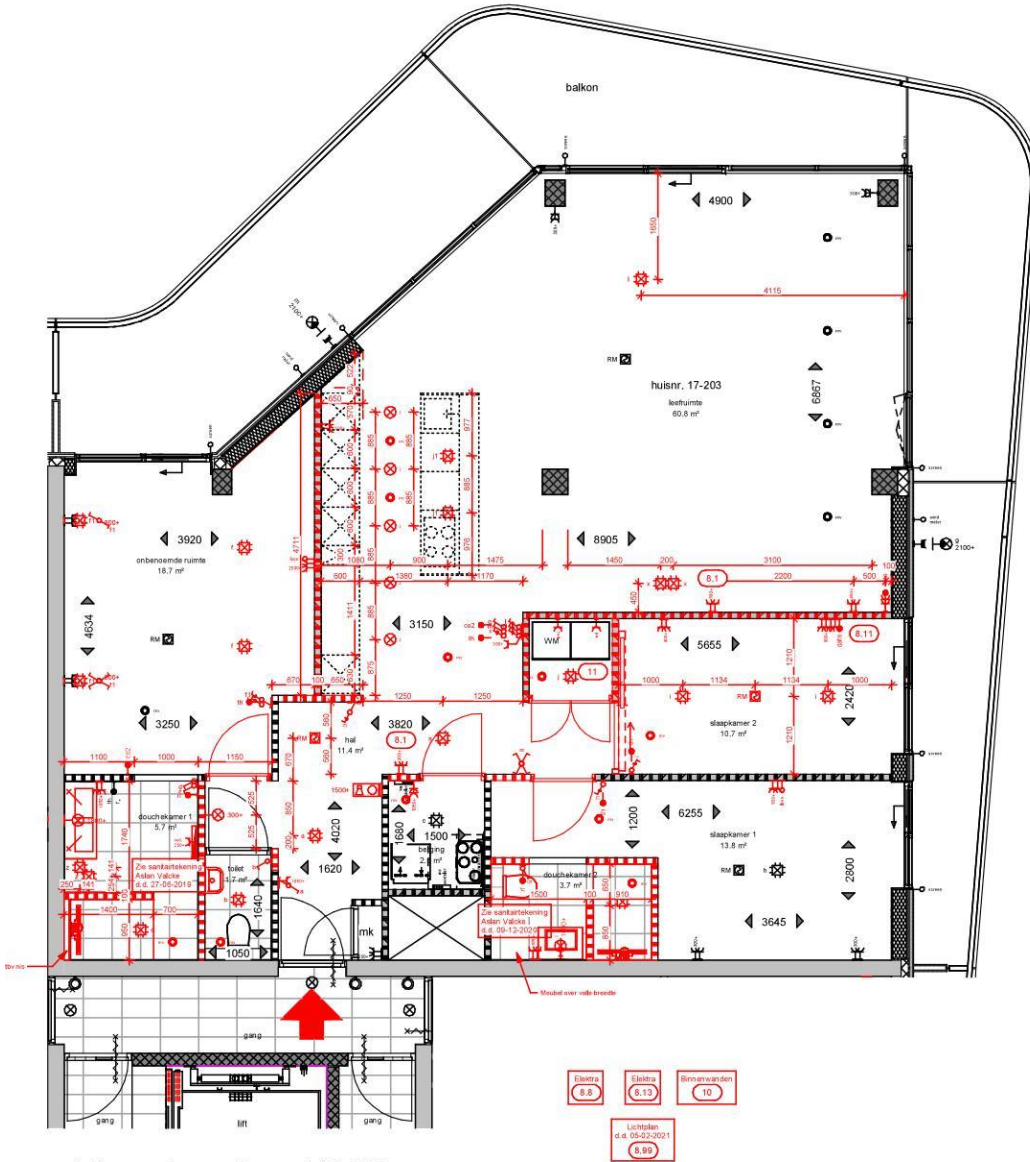
plattegrond appartement 17-203
