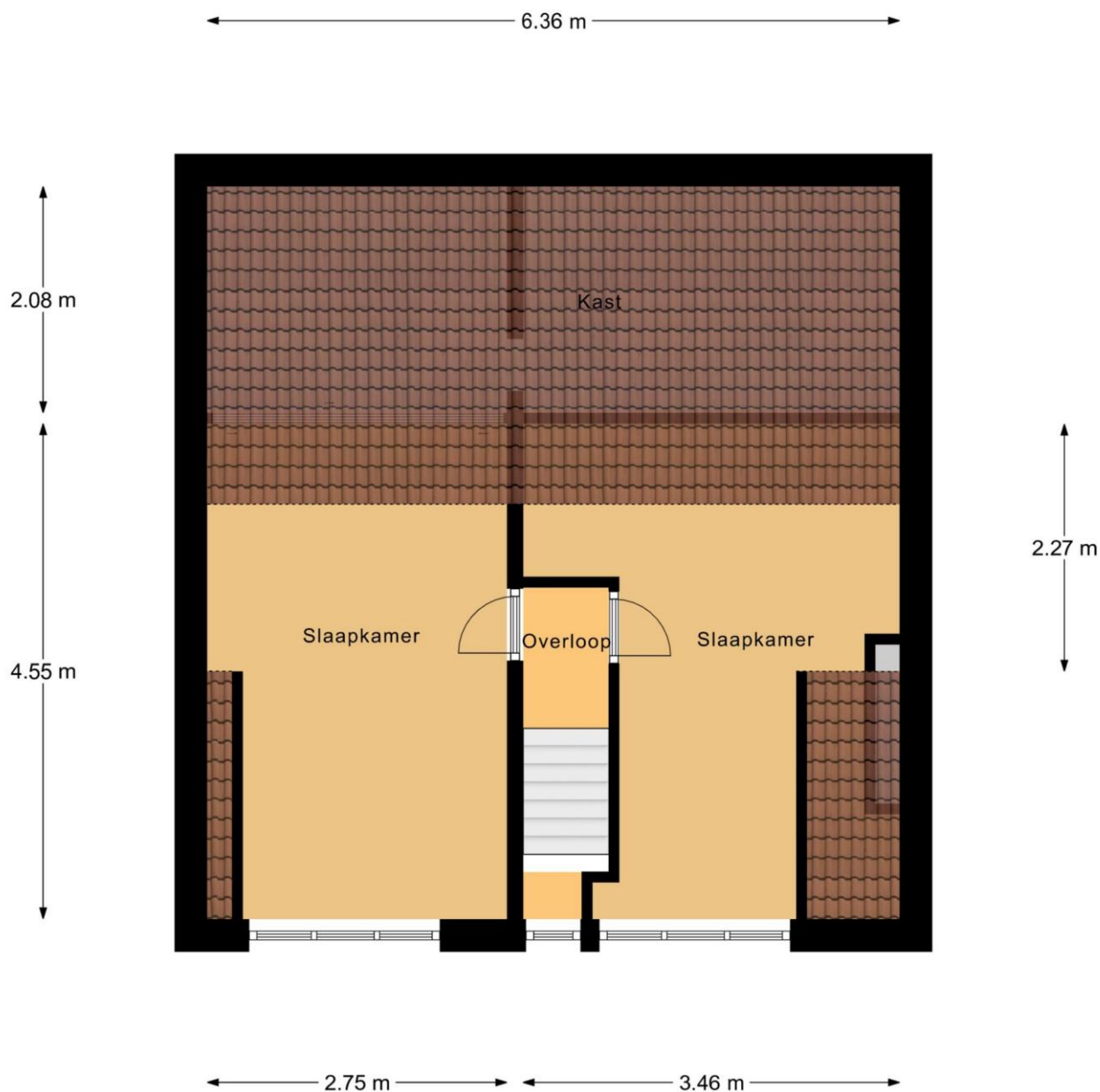
2e Verdieping
