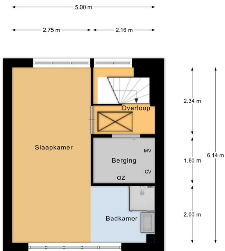
2e verdieping
