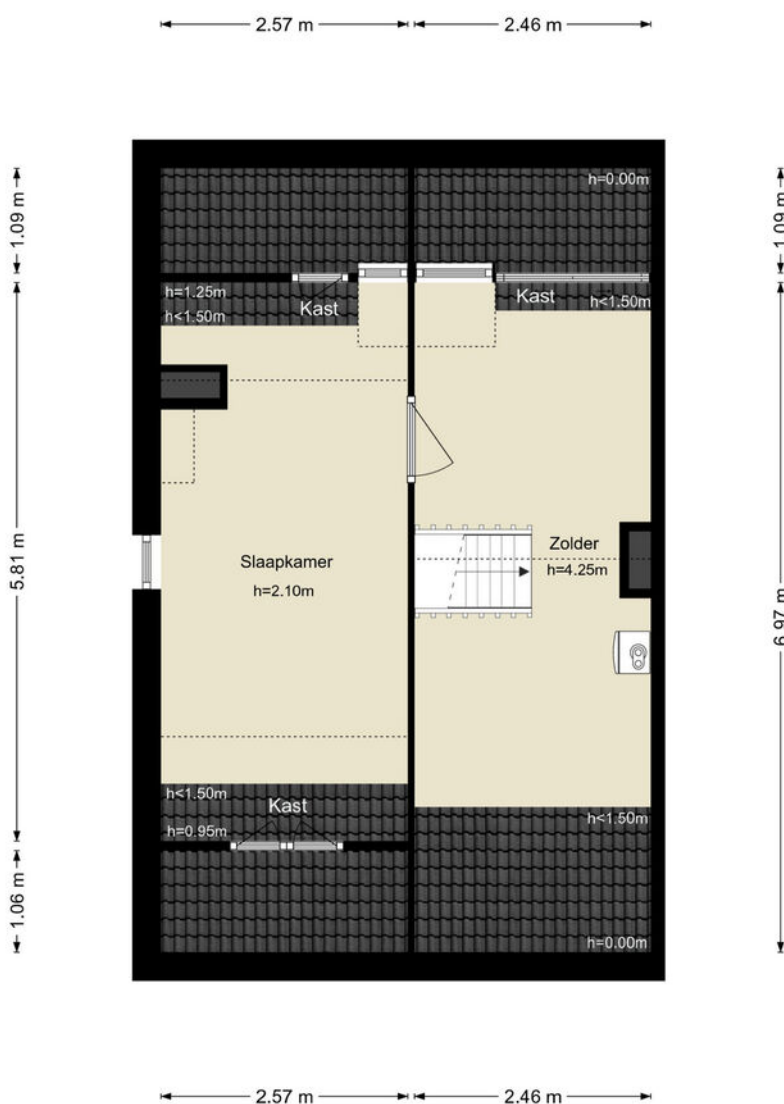
Meerndijk 78 - De Meern Tweede Verdieping
