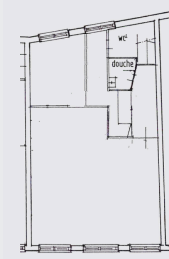
Eerste verdieping
