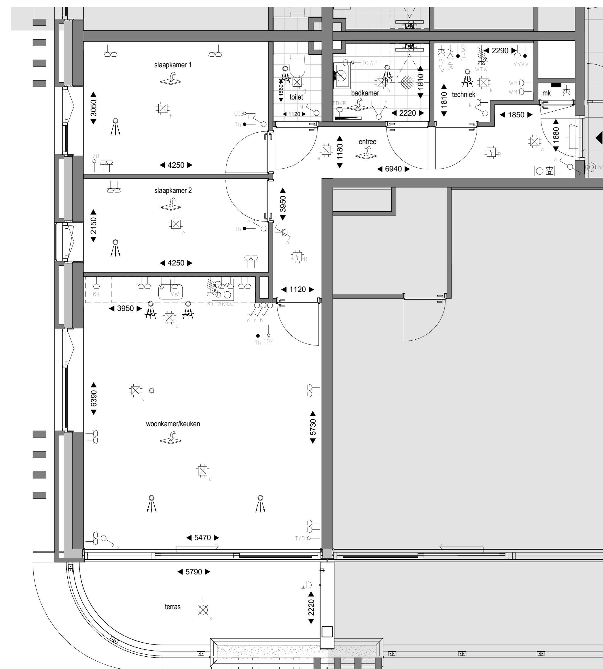
Plattegrond - bouwnummer 154 1: 50
