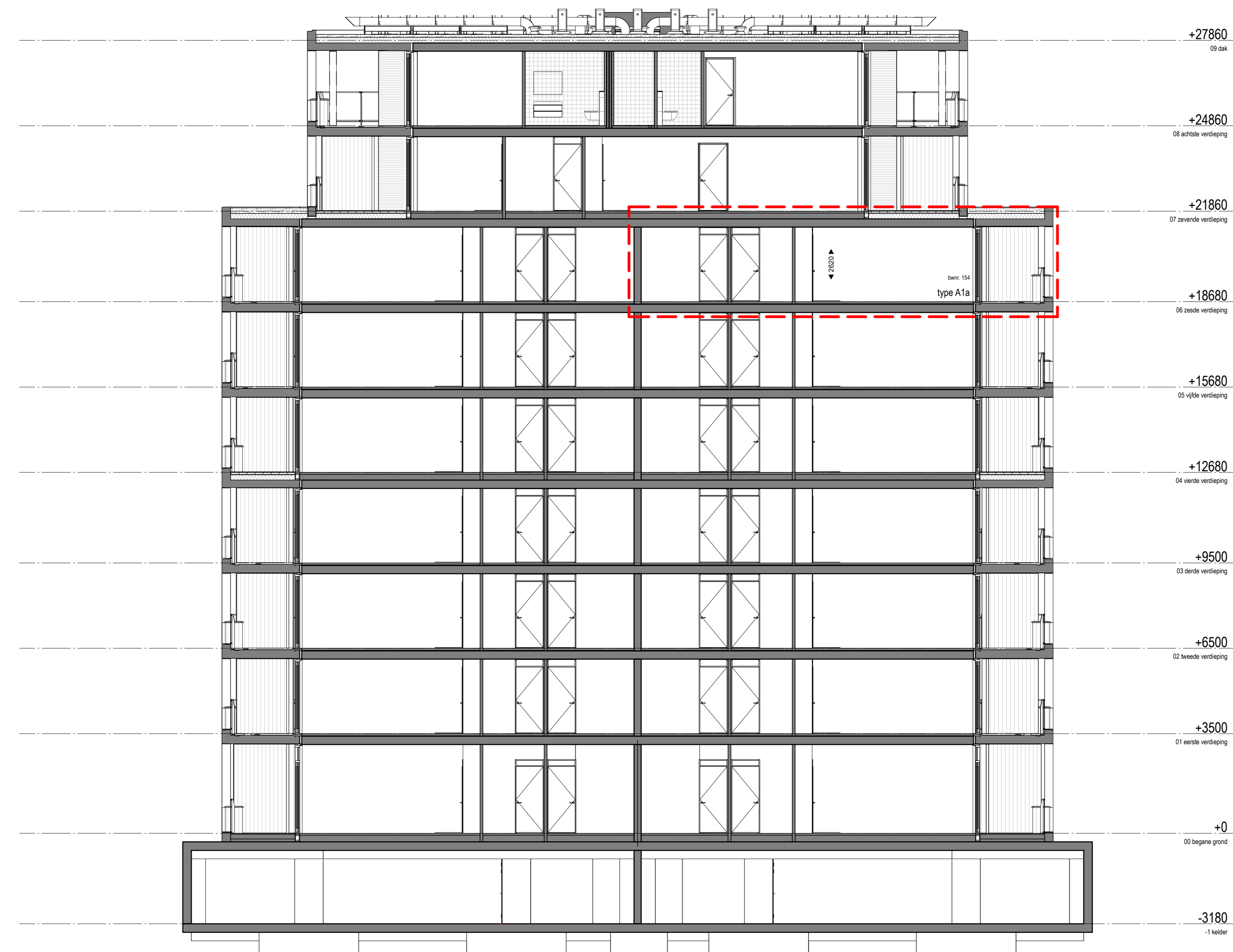
Doorsnede A - bouwnummer 154 1: 100
