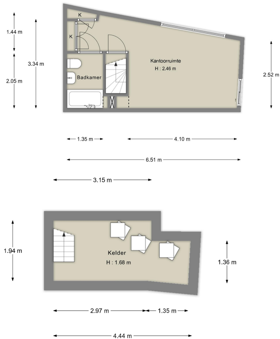
Kelder en eerste verdieping
