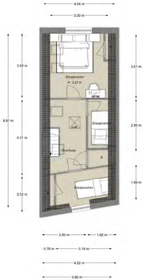
Eerste verdieping
