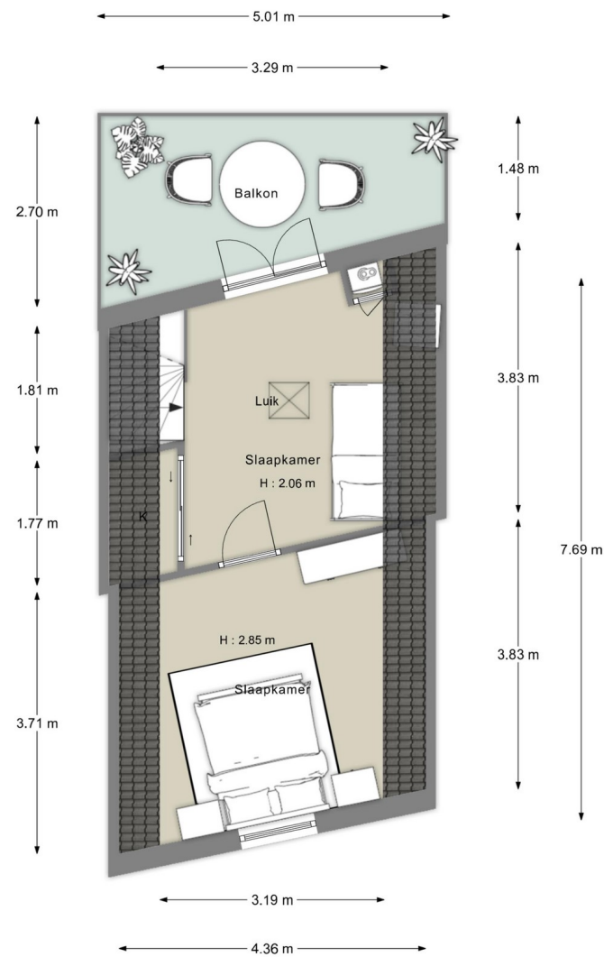
Tweede verdieping
