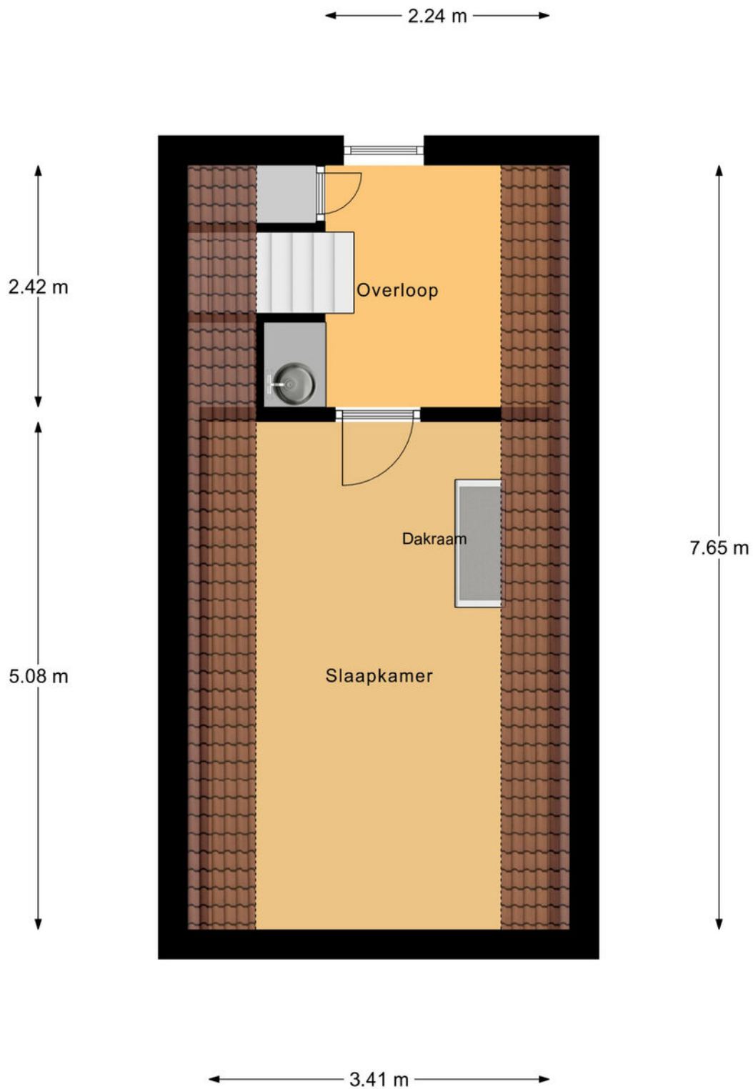
1e Verdieping-2
