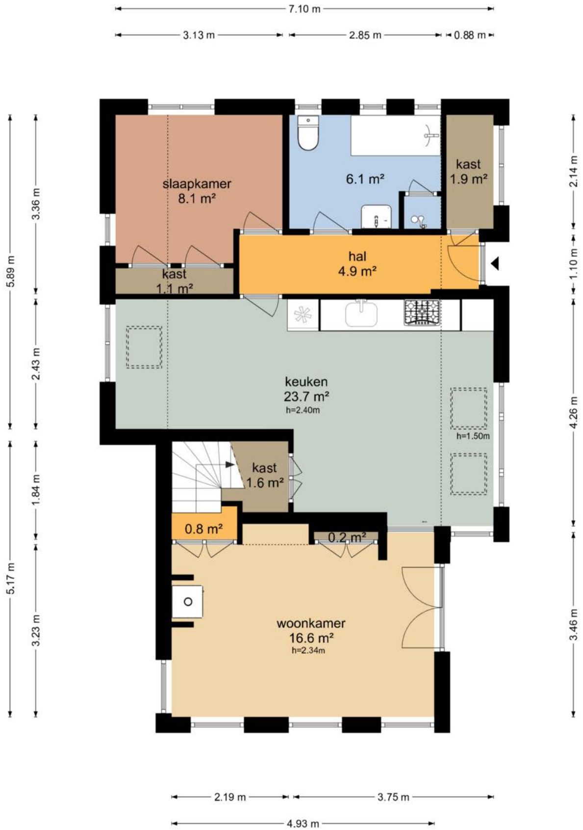
Begane grond
