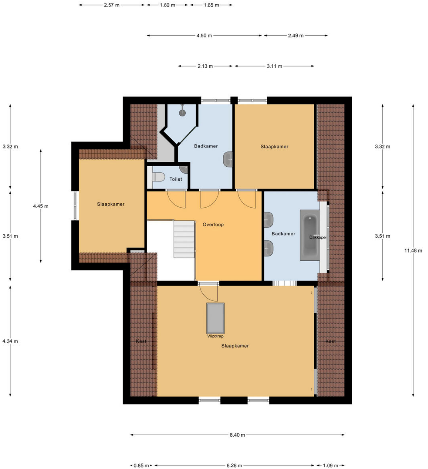
1e Verdieping
