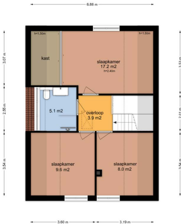
Eerste verdieping
