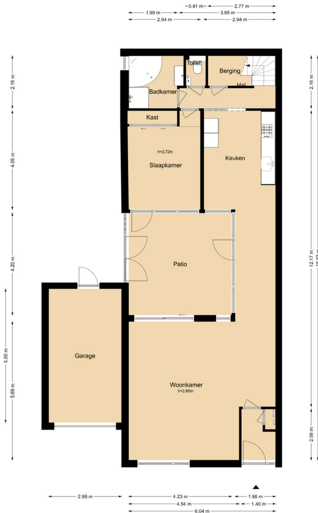
Begane Grond
