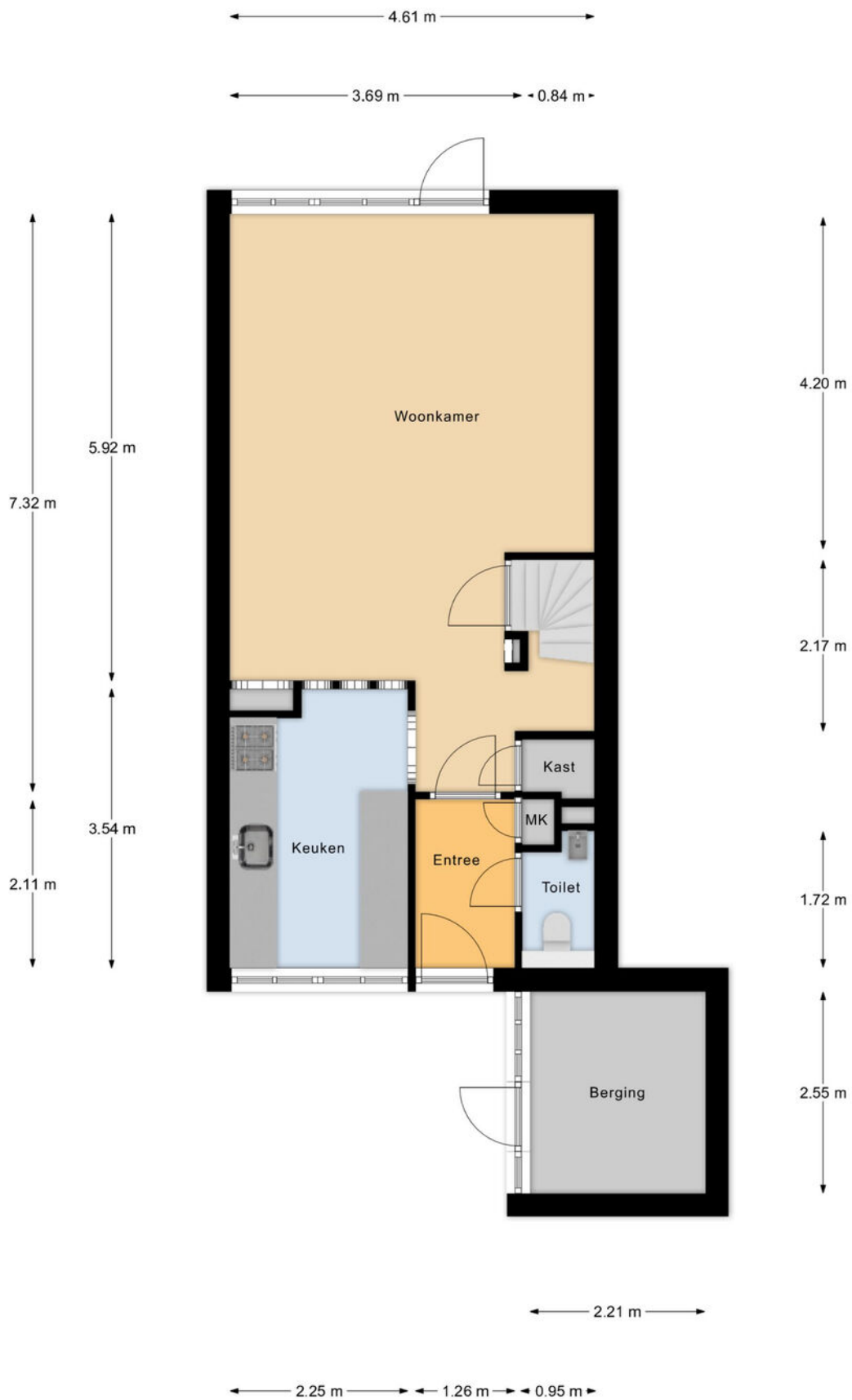
Begane Grond
