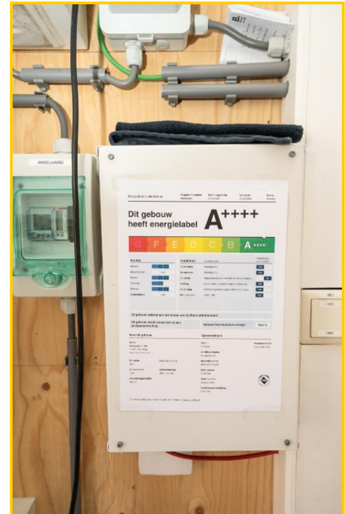
De groepenkast, het Watergenius wateroptimalisatiesysteem, de elektrameter, de watermeter en de omvormer zonnepanelen bevinden zich in de kastenwand aan de voorzijde van de showroom.
