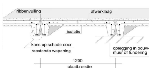
Figuur 2. Doorsnede Manta vloerelement
