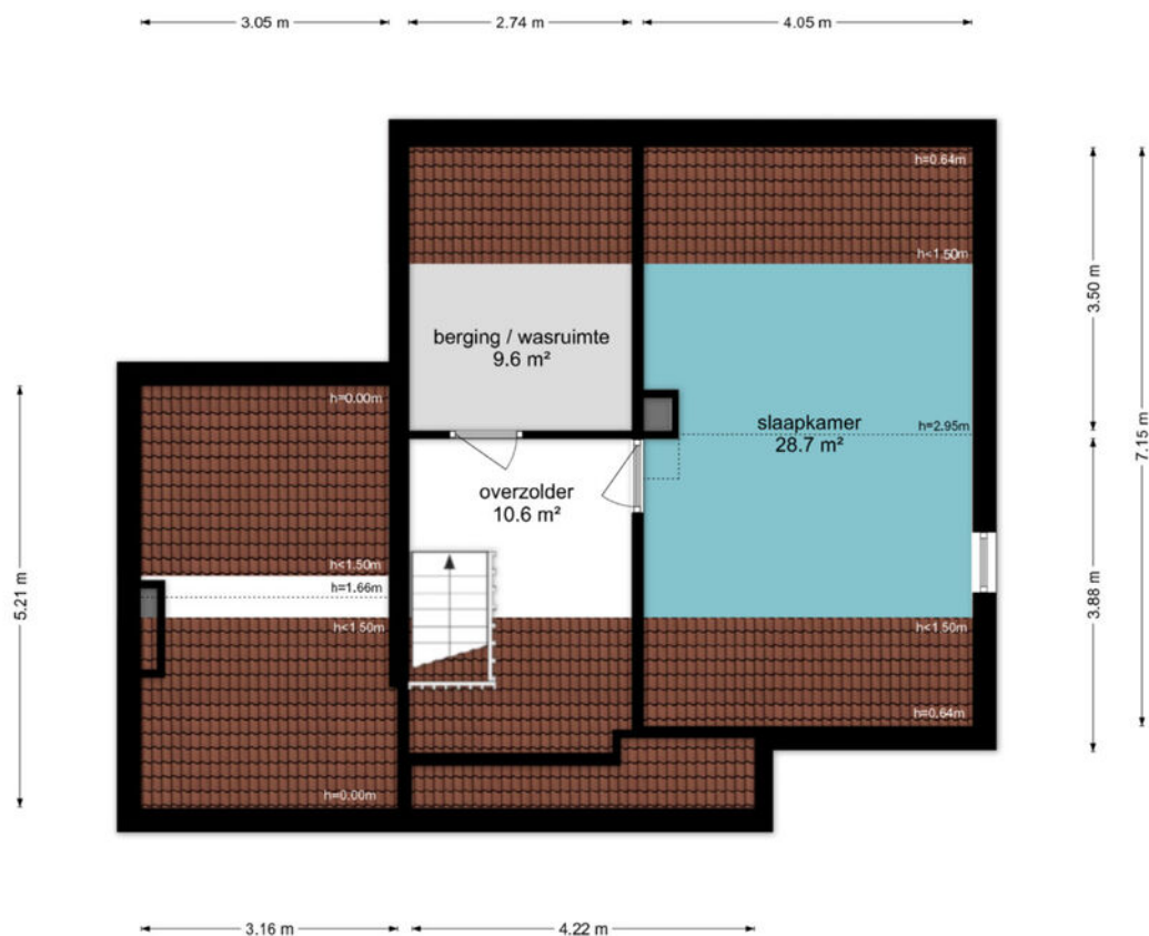
Langenakker 139 - Mierlo Tweede Verdieping
