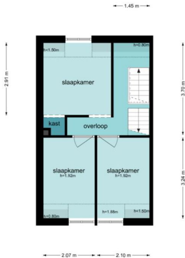
's Gravenwaardsedijk 27 - Tolkamer Eerste Verdieping
